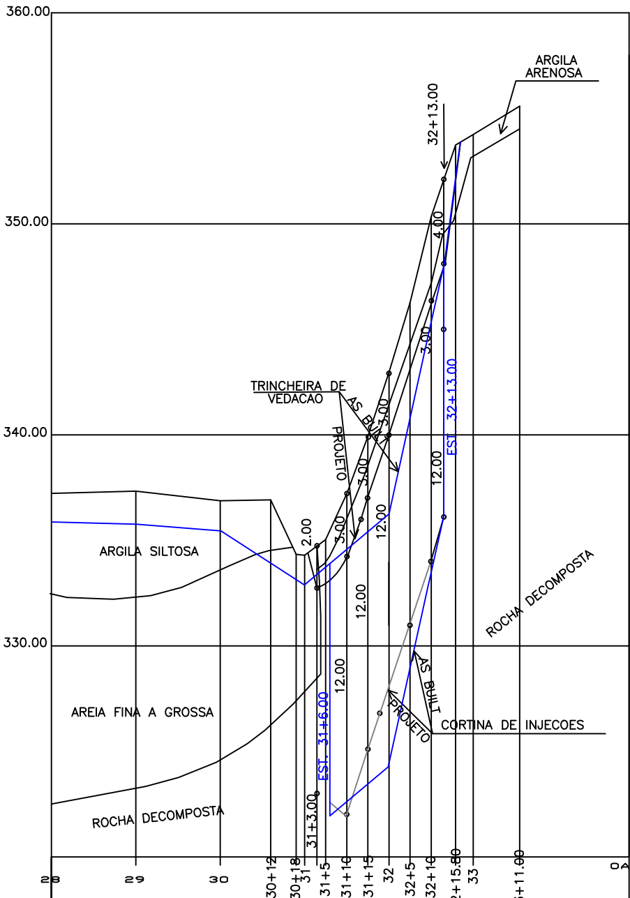
ZONA DE INJEÇÕES E TRINCHEIRA DE VEDAÇÃO PERFIL LONGITUDINAL ESC.: H: 1/1.250 V: 1/250
