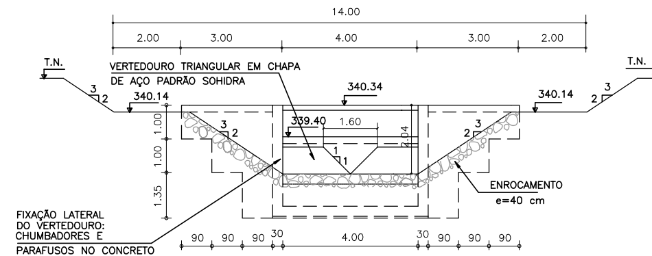
CORTE DD ESC.: 1/75
