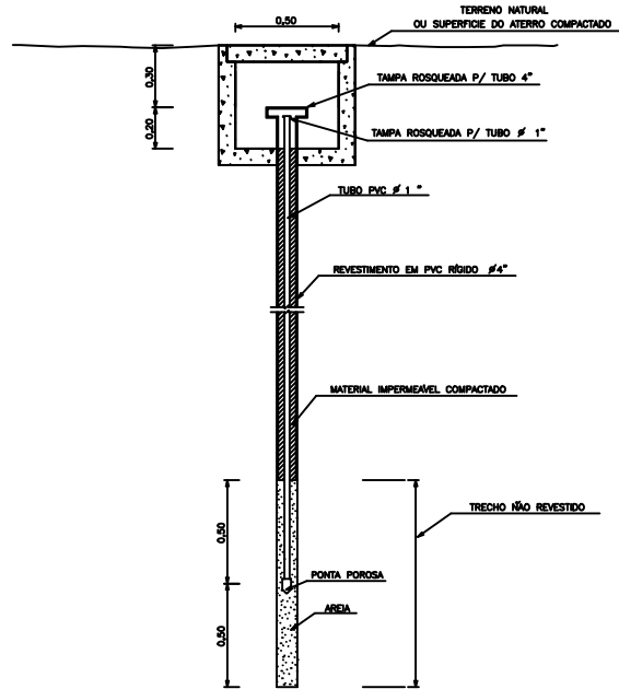
PIEZOMETRO ABERTO (TIPO CASAGRANDE) (LOCALIZADO NO MACICO E TERRENO NATURAL) ESC.: 1/20
