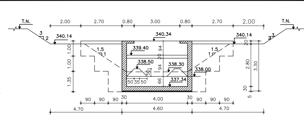
CORTE CC ESC.: 1/75
