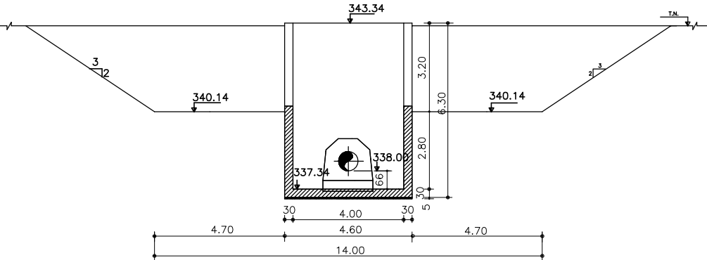
CORTE BB ESC.: 1/200
