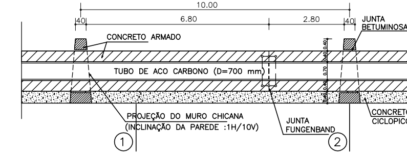
DETALHE DO ENVELOPAMENTO A MONTANTE ESC. 1/75
