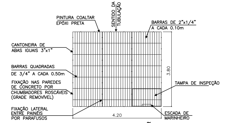
GRADE DE PROTEÇÃO DA CAIXA DE VÁLVULAS (3 MÓDULOS REMOVÍVEIS) ESC.: 1/100
