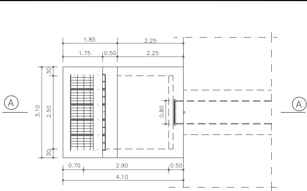
OBRA DE MONTANTE ESC.: 1/100
