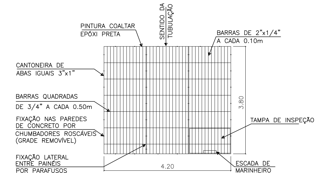
GRADE DE PROTEÇÃO DA CAIXA DE VÁLVULAS (3 MÓDULOS REMOVÍVEIS) ESC.: 1/100
