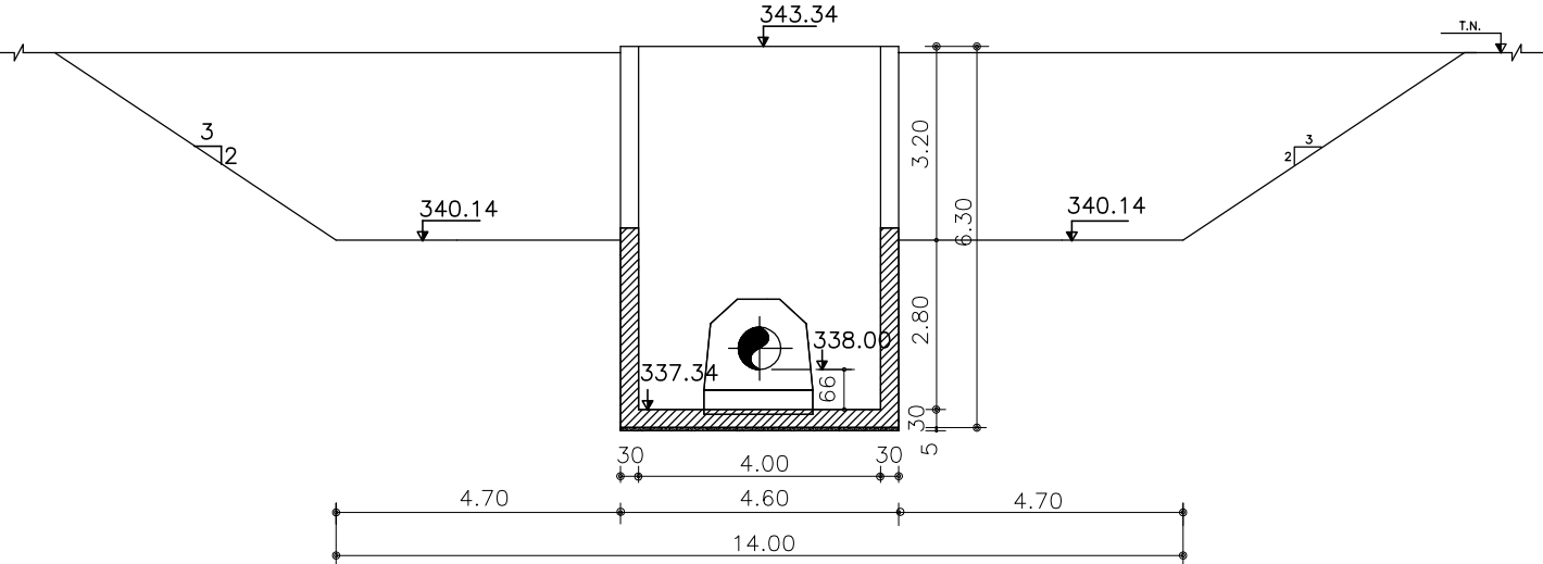
CORTE BB ESC.: 1/200
