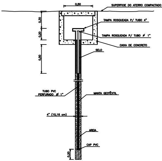
MEDIDOR DE NÍVEL D'ÁGUA ESC.: 1/20
