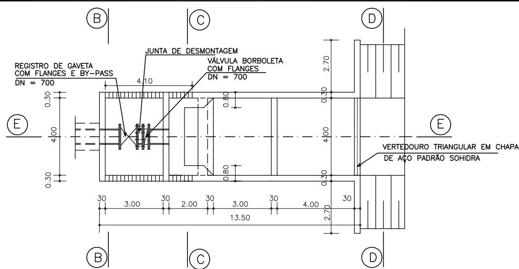
OBRA DE JUSANTE - PLANTA ESC.: 1/200
