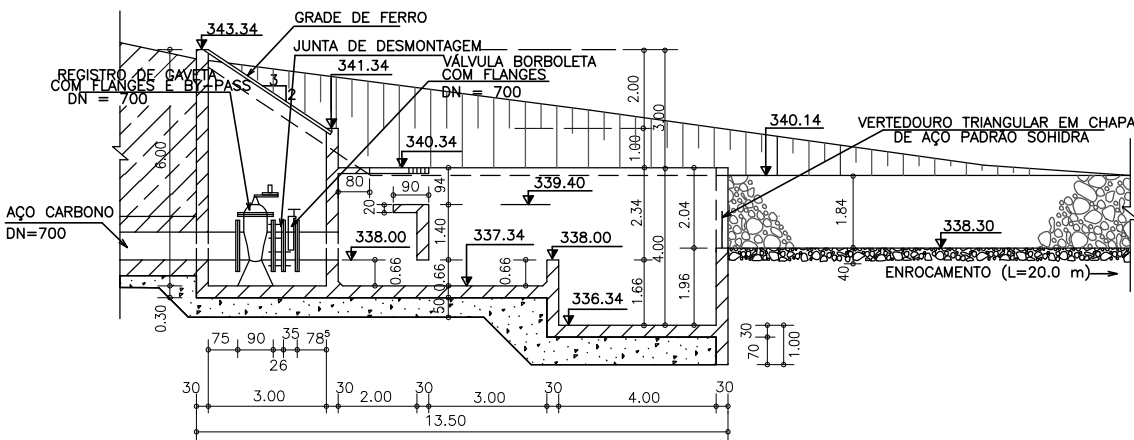
CORTE EE ESC.: 1/200
