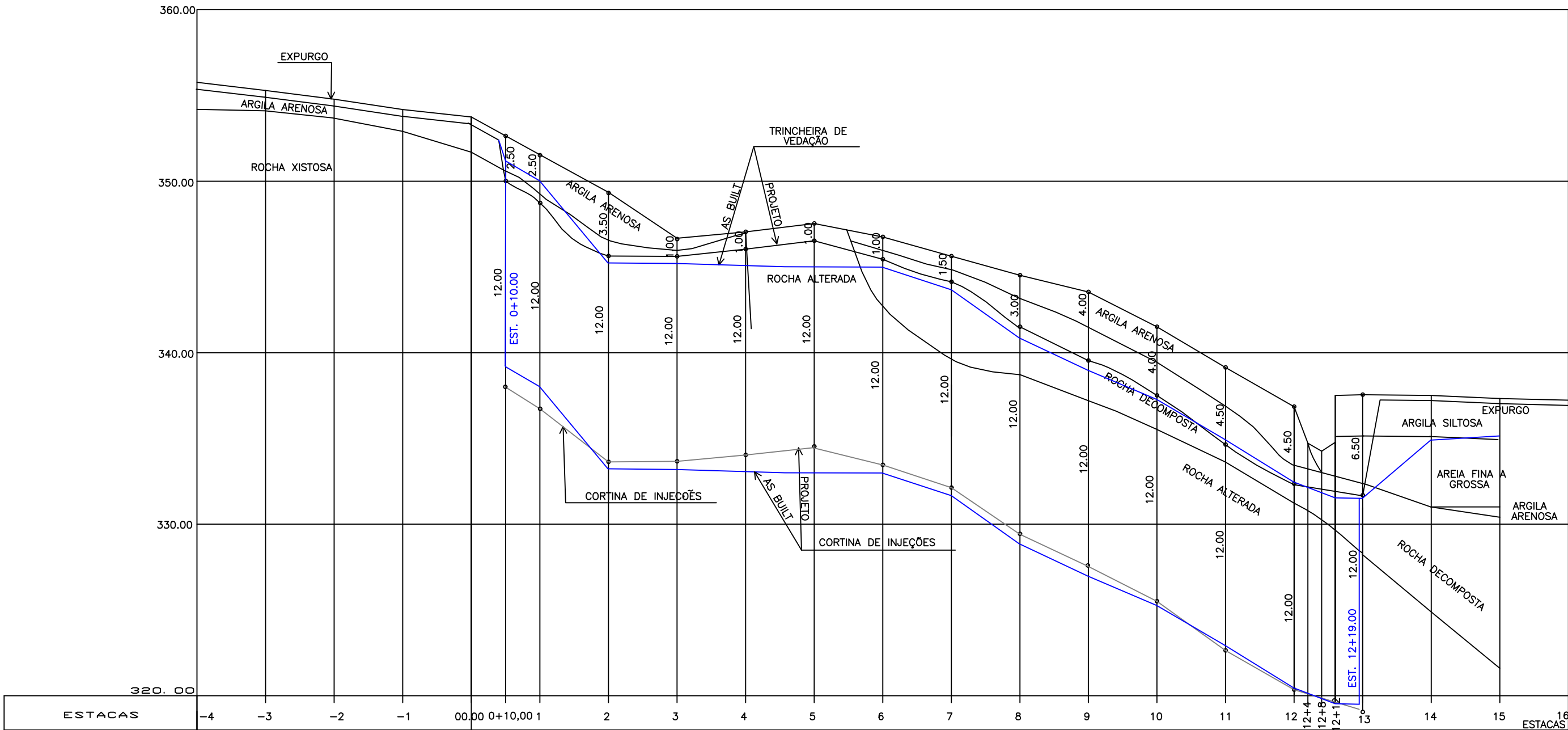
ZONA DE INJEÇÕES E TRINCHEIRA DE VEDAÇÃO PERFIL LONGITUDINAL ESC.: H: 1/1.250 V: 1/250
