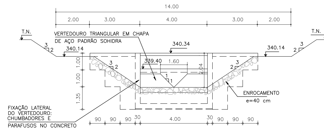
CORTE DD ESC.: 1/75
