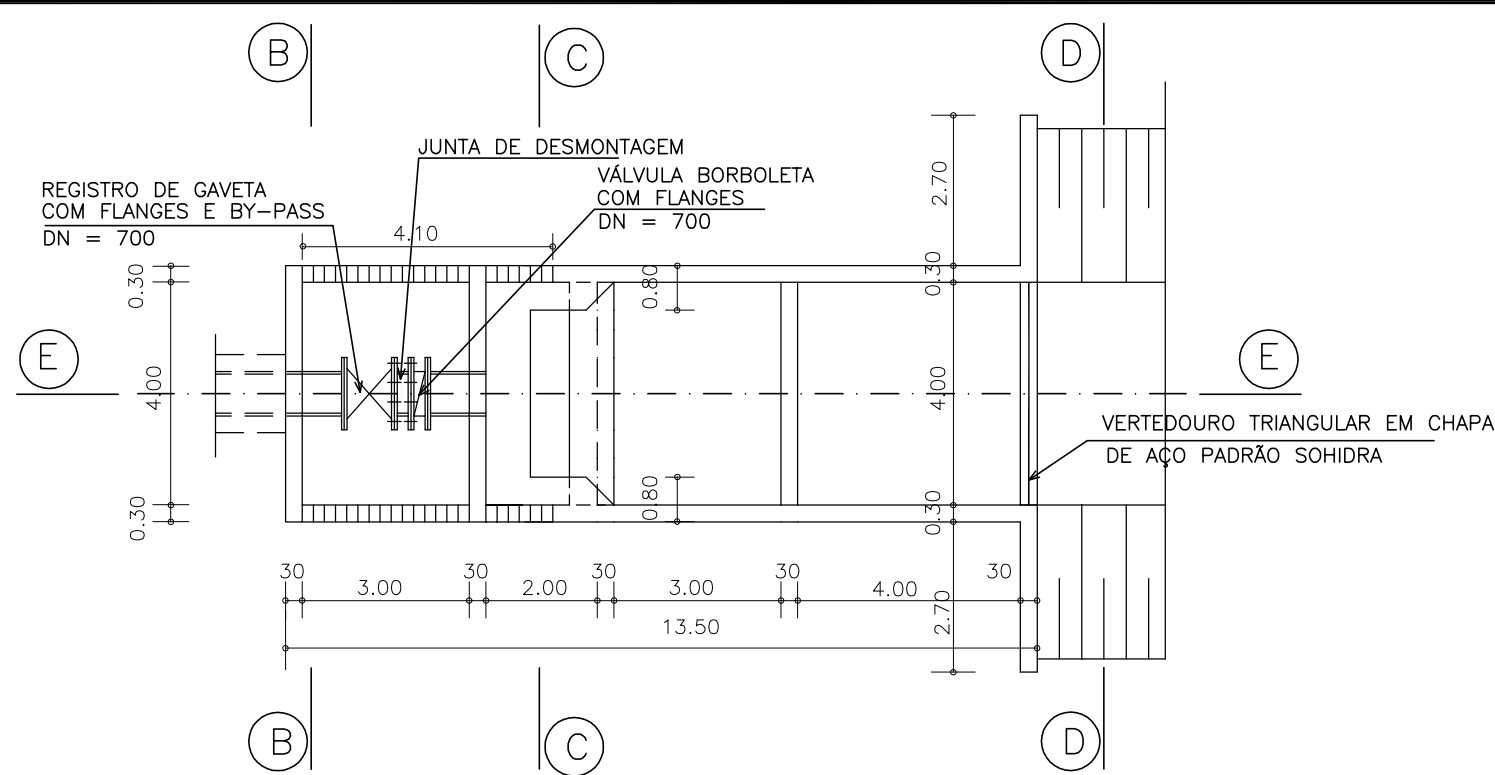
OBRA DE JUSANTE - PLANTA ESC.: 1/200
