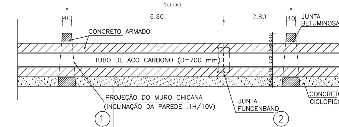
DETALHE DO ENVELOPAMENTO A MONTANTE ESC. 1/75
