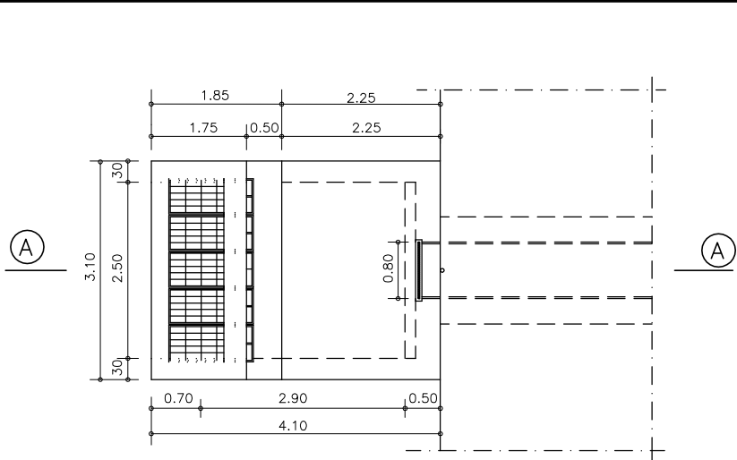
OBRA DE MONTANTE ESC.: 1/100
