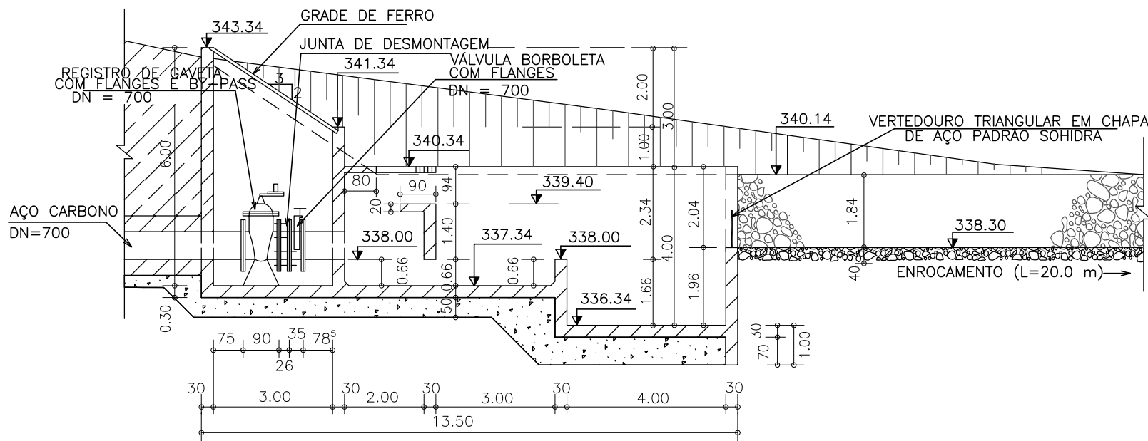
CORTE EE ESC.: 1/200
